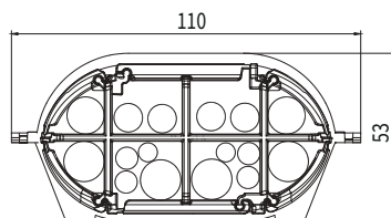
(2)带一体式分线器
