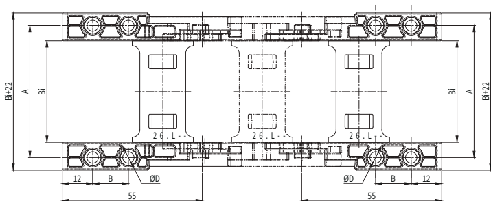
拖链示意图 Cable chain diagram
