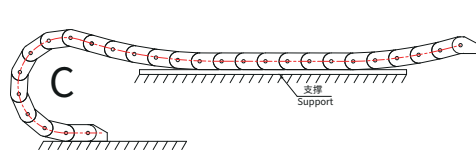
FLB区的支撑 C) 最长可增加100%行程
