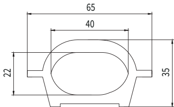
(1)标准款允许最多安装管线： 6根φ7~φ8 +4根φ4~φ6
