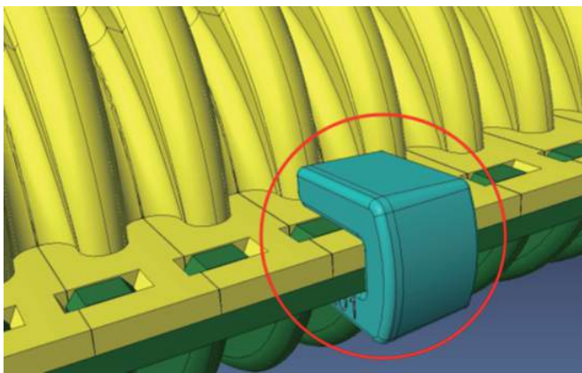
卡扣WZ.015 Clip WZ.015
