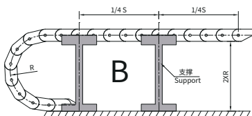
FLG区域支撑 B)增加100%的直线架空距离
