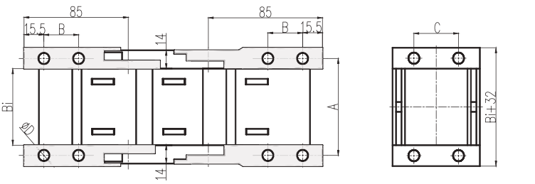
拖链示意图 Cable chain diagram
