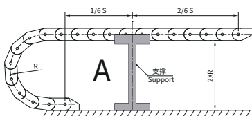
FLG区域支撑 A)此类可以增加50%的直线架空距离
