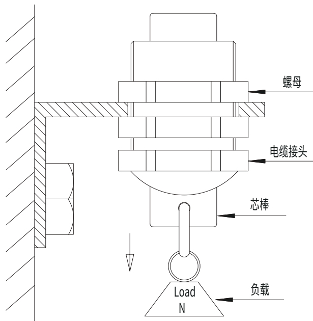
电缆接头夹紧拉力测试
