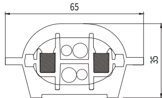
(3)带轻型龙骨允许最多安装 管线:2根φ6~φ7 +2根φ4~φ5
