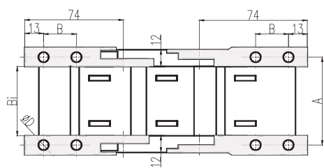
拖链示意图 Cable chain diagram
