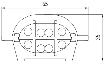
(2)带横竖隔片允许最多安装 管线:4根φ6~φ7 +4根φ4~φ5 ★横竖隔片建议12组/米
